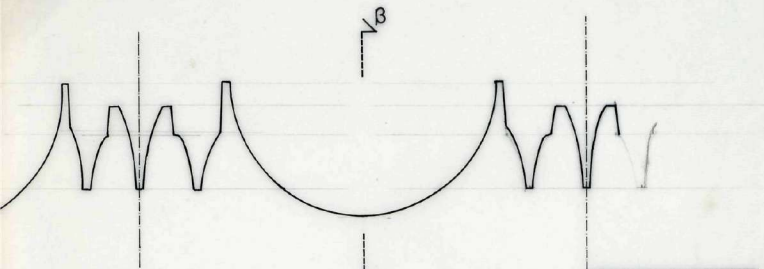
τομή α-α 1:1 υπαρκτούα κατάσταση
